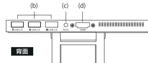
(b) USB-A 2.0 x3 (カメラ、タッチスクリーン、マウスやキーボード などのアクセサリ接続用)
